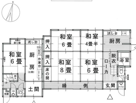
1階間取図
